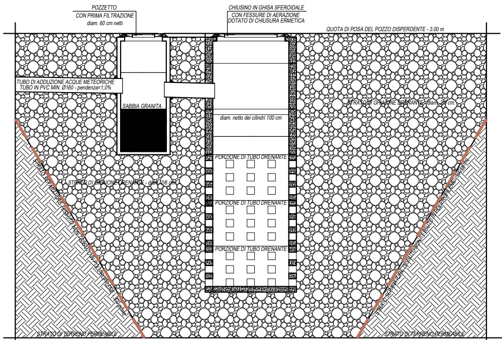
DETTAGLIO POZZO DISPERDENTE scala 1:50
