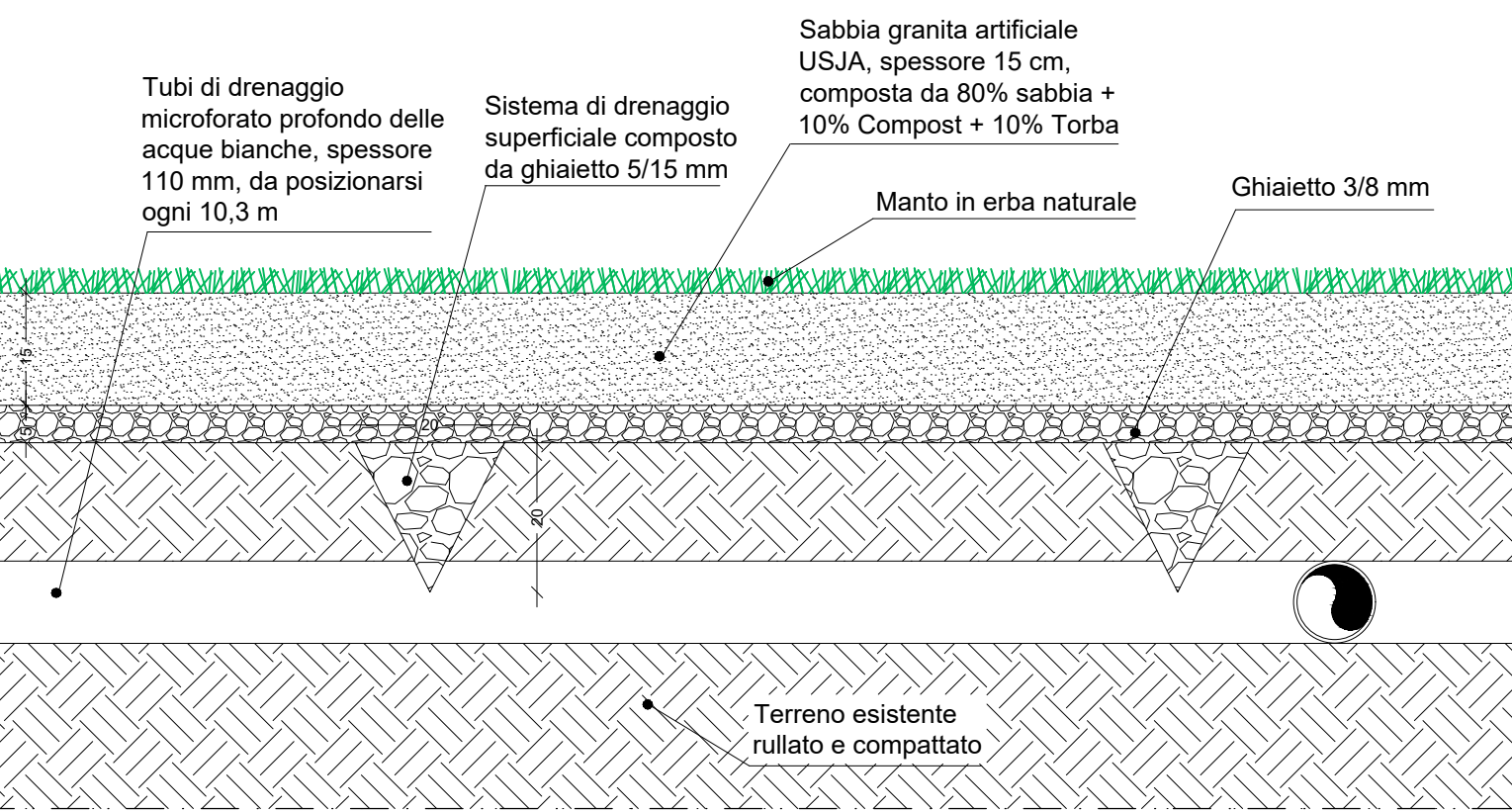
DETTAGLIO PAVIMENTAZIONE CAMPO scala 1:10
