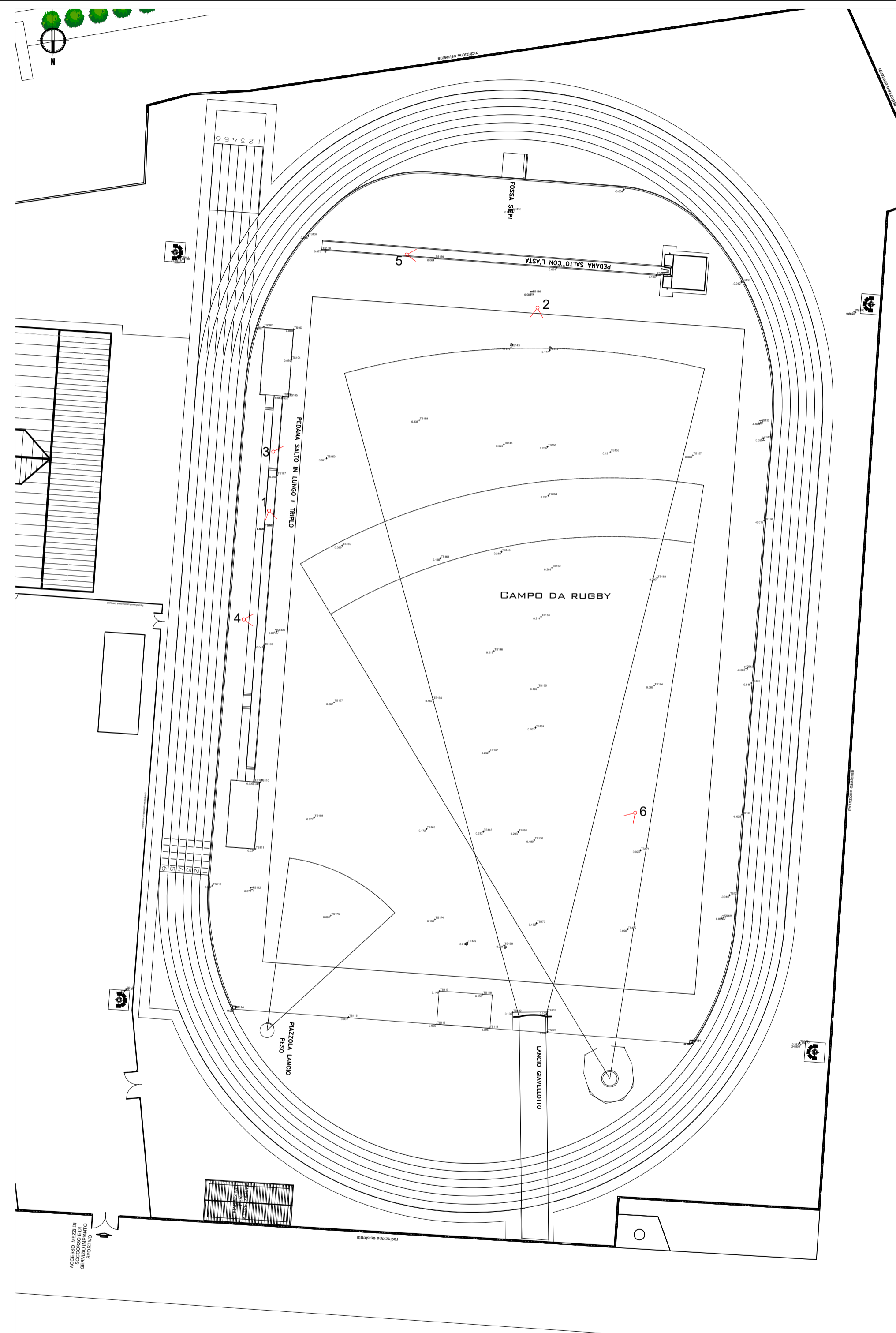
PLANIMETRIA CON RILIEVO STRUMENTALE scala 1:500
