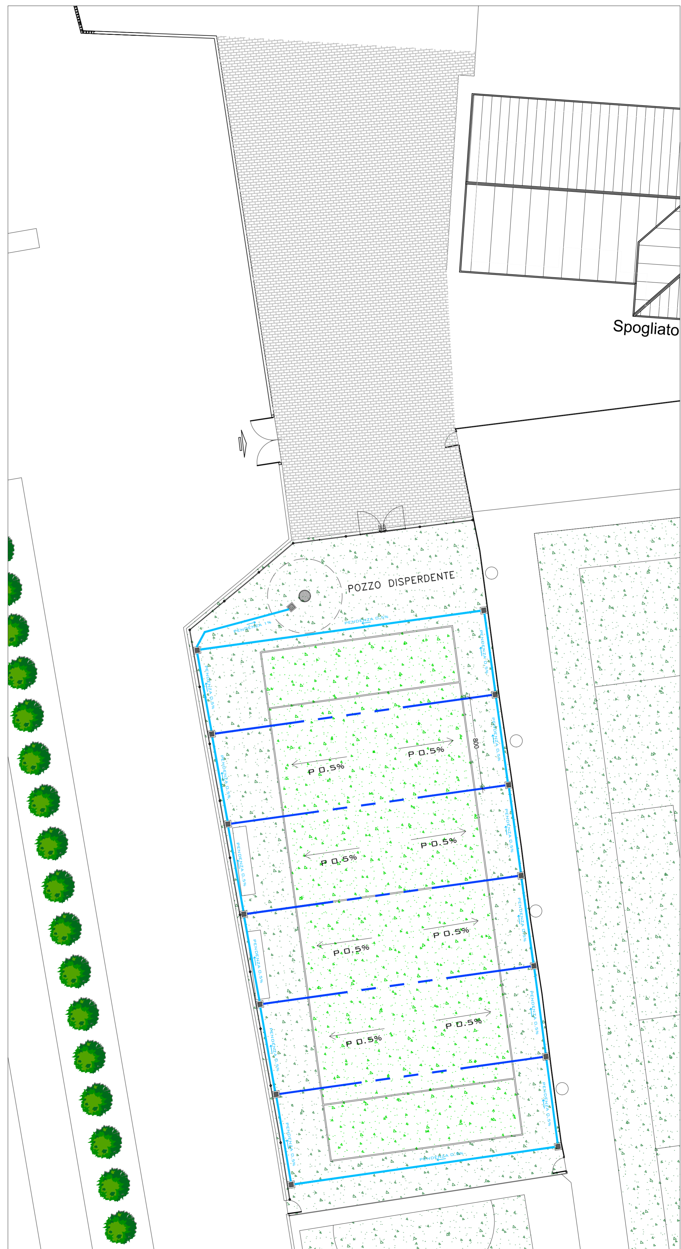
PLANIMETRIA SISTEMA DI DRENAGGIO scala 1:200
