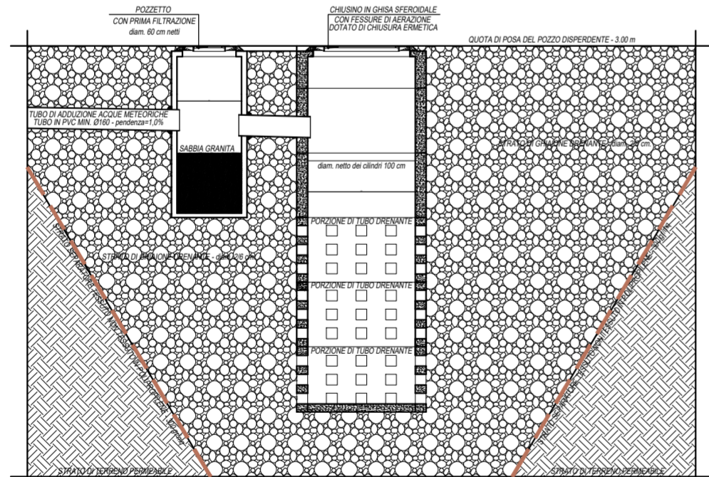
DETTAGLIO POZZO DISPEDENTE scala 1:50
