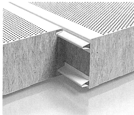
Fig. 1 - particolare del pannello SIL-Modular®
